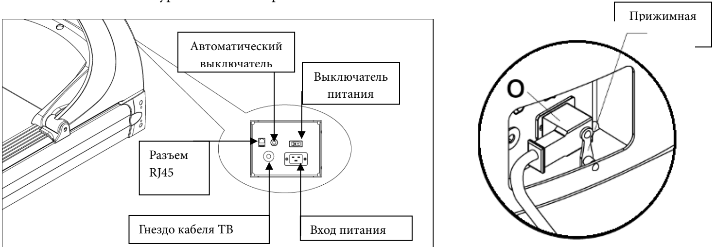
Рис. 11-1. Передняя электрическая панель беговой дорожки CS900 (показана панель на 120 В)
